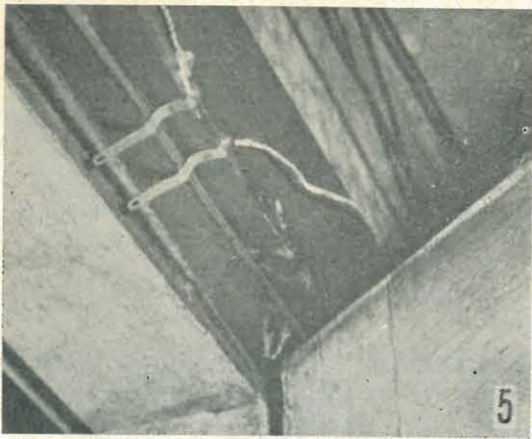
Sistema di rilevamento di allarme per la porta di un garage. Se la chiusura del garage o della rimessa è del tipo a serranda avvolgibile, conviene fare ricorso al sistema del filo a zig-zag, sistemato all'interno.
