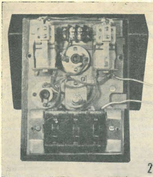
Veduta interna del complesso centrale: in basso gli interruttori a levetta, poco sopra, il pulsante, a fianco, il portalampane per una delle lampadine, sopra, la lampadina, in serie alla prima, ma che serve da spia; in alto, ai lati i due relays, al centro, in alto, una morsettiere.
