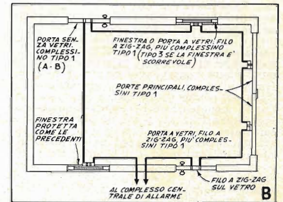
Circuito tipico, per la protezione di un certo numero di porte e di finestre: lo stesso circuito vale, sia per l'edificio principale, sia per una costruzione indipendente da quest'ultimo.
