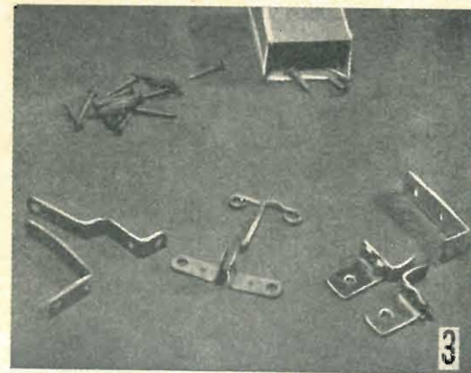
In questa foto sono illustrati alcuni tipici complessi, per il rilevamento di un tentativo di effrazione. I chiodini in alto a sinistra, servono per sostenere il filo a zig-zag, delle finestre e delle porte a vetri; in basso, a sinistra, al centro, a destra, sono delle coppie di contatti da fissare a parti mobili, in modo che quando una delle parti viene allontanata dall'altra, l'allarme entri in funzione. Nel disegno a lato la dimostrazione delle varie applicazioni.
