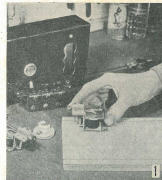
Studio della disposizione delle varie parti del pannello di supporto, in funzione della forma e delle dimensioni di ciascuna parte; la bassetta, in questo caso è di semplice legno, ben secco.
